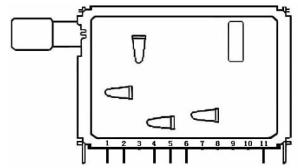
2+3+1 脚电压合成高频头
