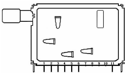
6+1 脚电压合成高频头
